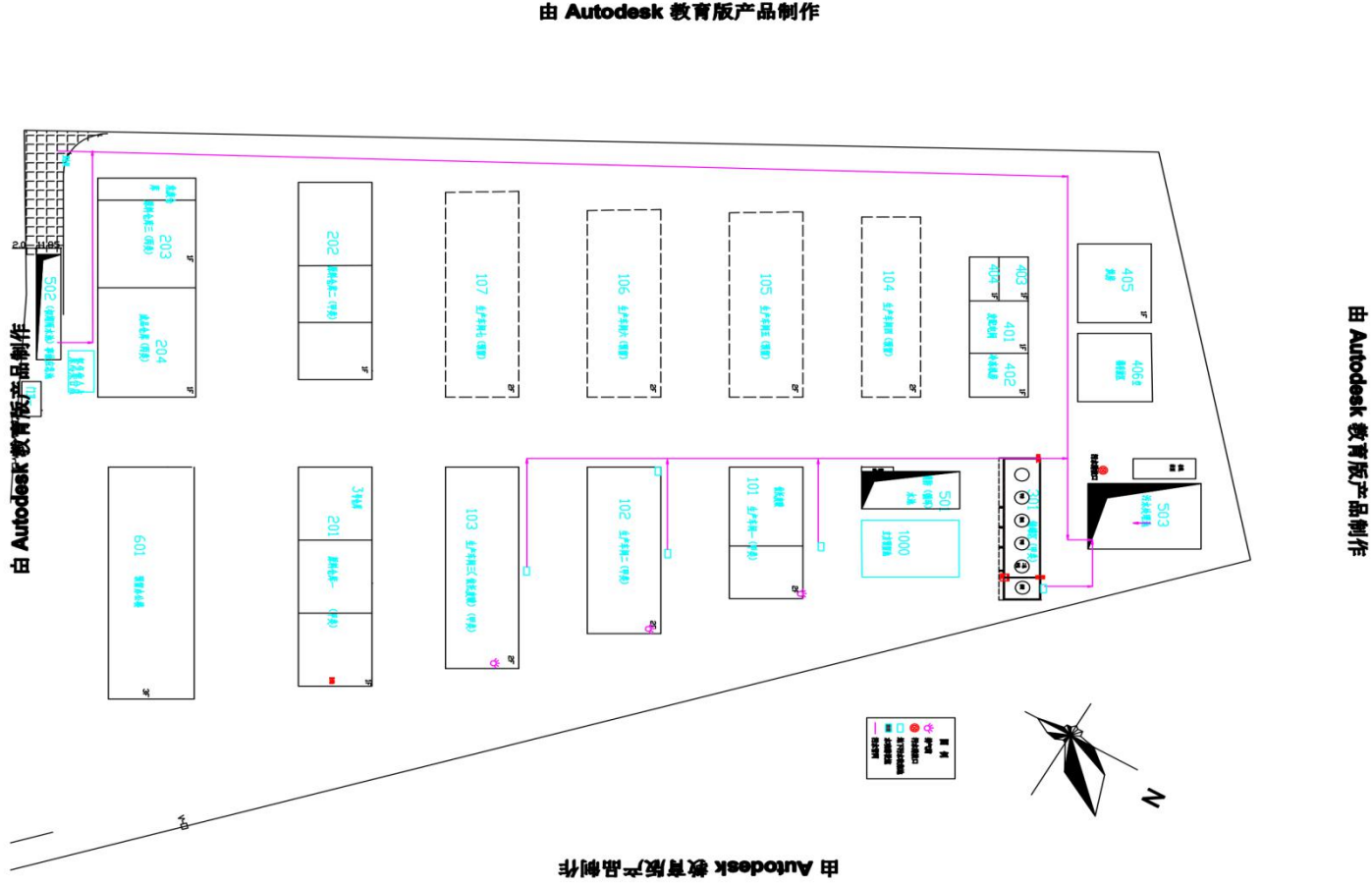
附图 5 企业污水管网图
